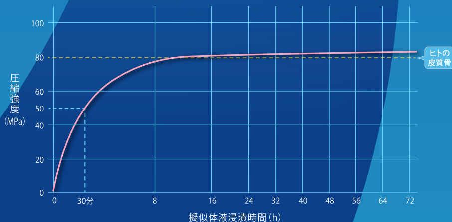
■ 補填後72時間までの圧縮強度
